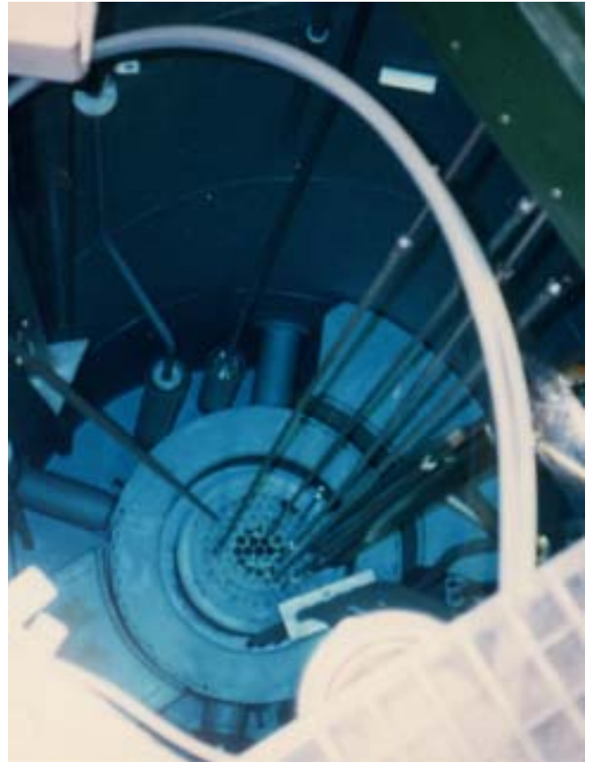
小型原子炉の炉心．青く見えるのは放射線が水を通るときに出るチェレンコフ光．（ウーン大学）
